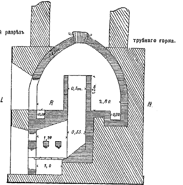
Г. Для трубногo горна 1 мет. въ 1 с/м.
