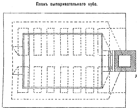
Планъ выпаривательнаго куба.
